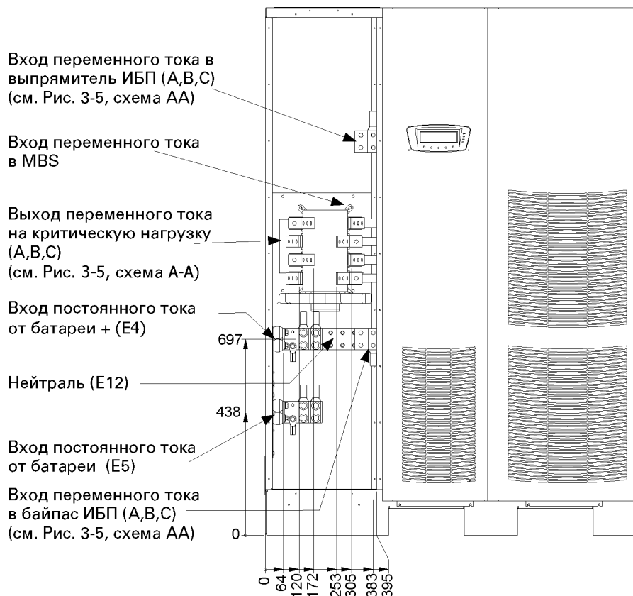
Рис. 3-4. Местоположение силовых клемм ИБП
