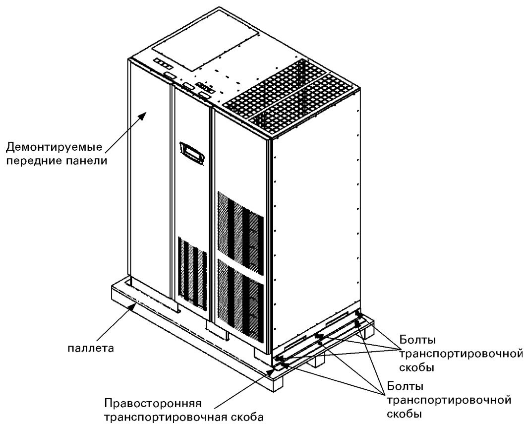
Рис. 3-2. Демонтаж правой транспортировочной скобы
