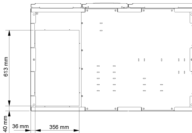
Рис. 2-4. Размеры ИБП (вид снизу)
