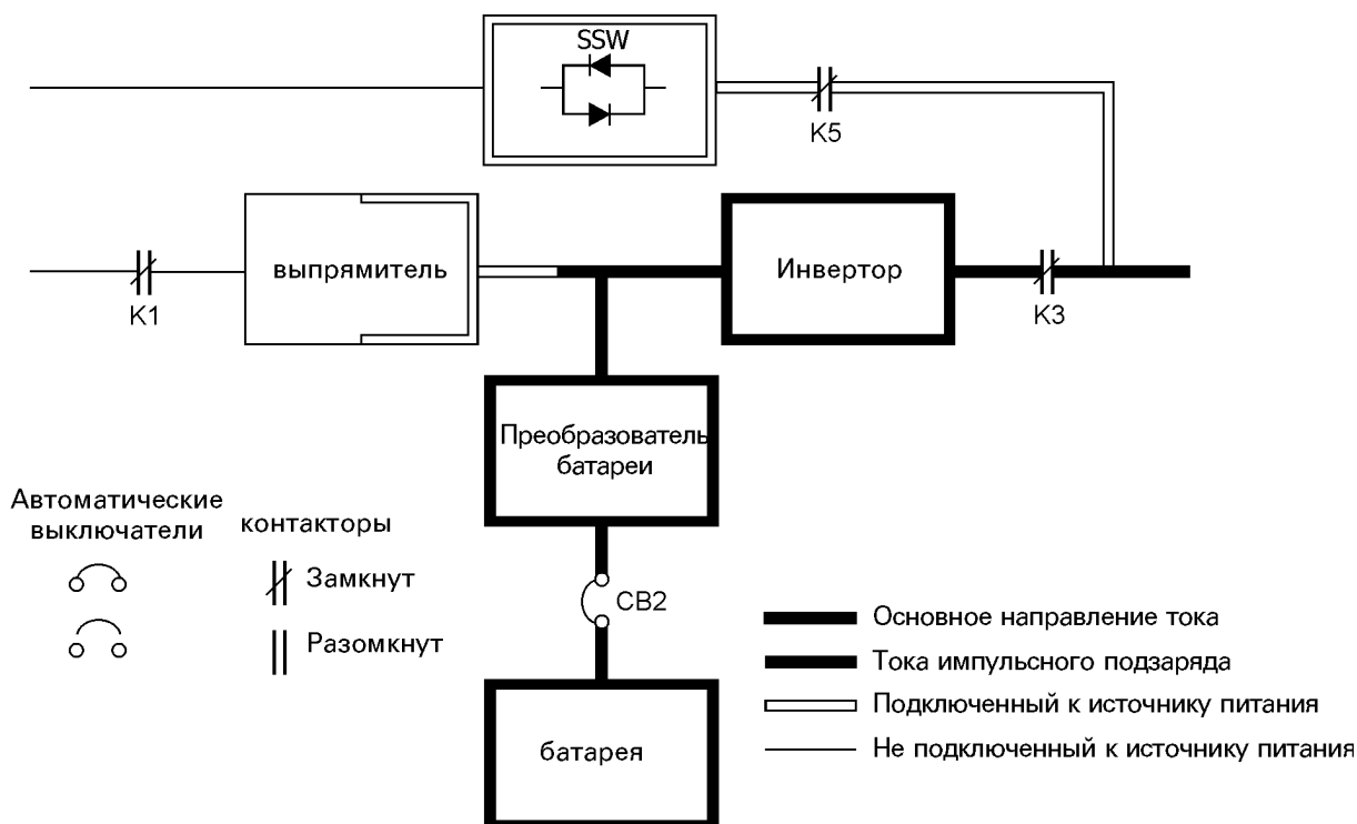
Рис. 4-4. Путь электрического тока через систему ИБП во время ее работы в режиме работы батарей
