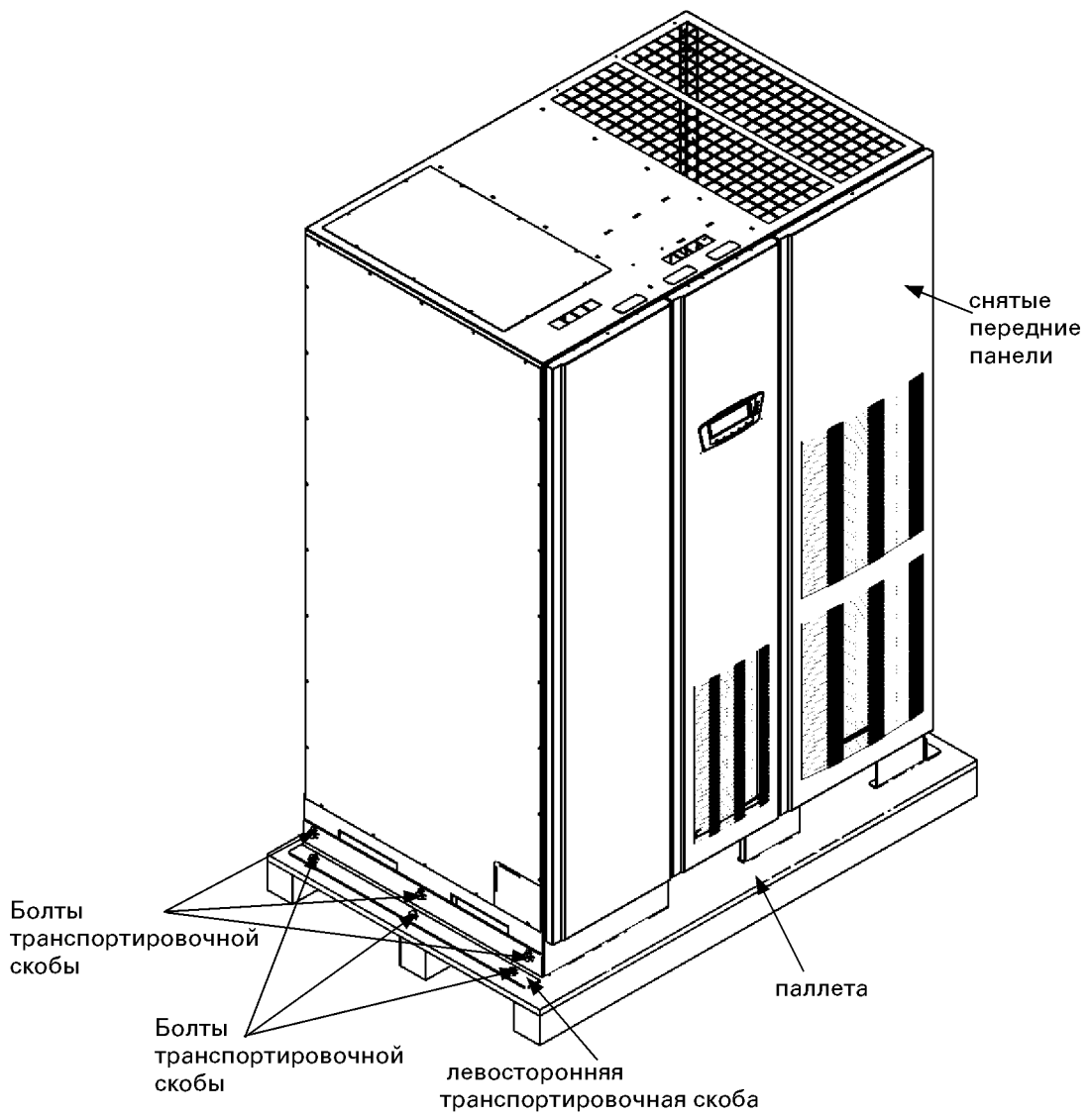
Рис. 3-1. Демонтаж левой транспортировочной скобы
