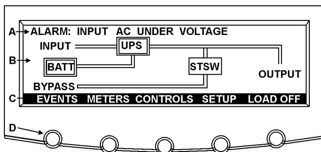
Рис. 5-3. Зоны ЖК-дисплея.
