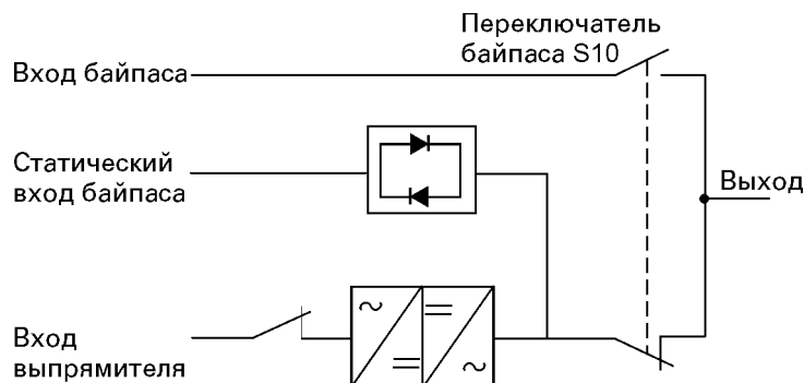
Рисунок 5-8. Типовое расположение MBS переключателей и переключатель для отключения выпрямителя (должен быть размещен на данном участке).
