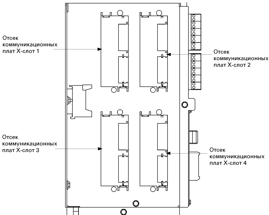
Рис. 3-11. Коммуникационные отсеки плат X-Слот
