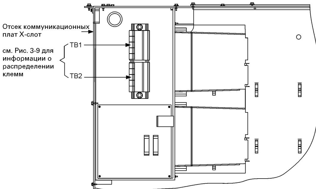
Рис. 3-8. Схема клемм подключения внешних устройств АА
