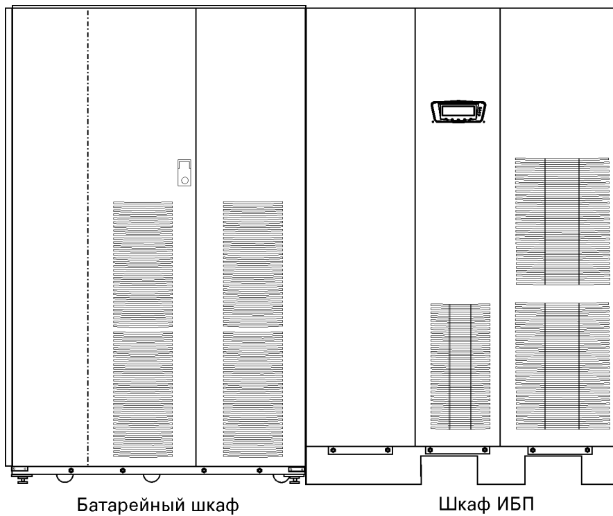
Рис. 1-2. Стандартная система ИБП Powerware 9395 (225–275 кВА)
