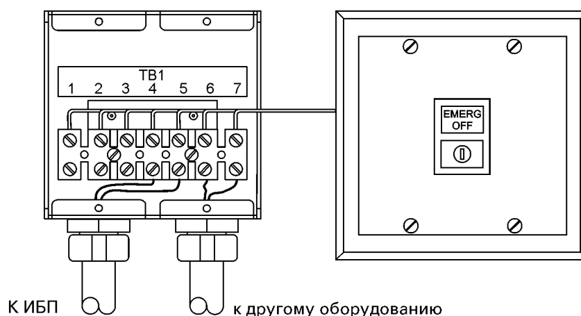
Рис. 3-12. выключатель дистанционного аварийного отключения ИБП
