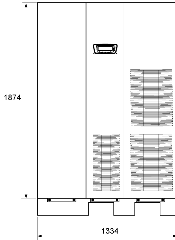
Рис. 2-1. Размеры ИБП (вид спереди)
