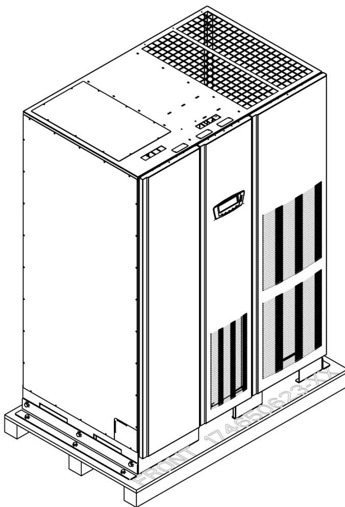
Рис. 2-8. Шкаф ИБП Powerware 9395 (225–275 кВА) при транспортировке на поддоне
