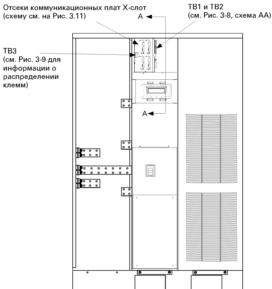
Рис. 3-7. Расположение клемм для подключения внешних устройств
