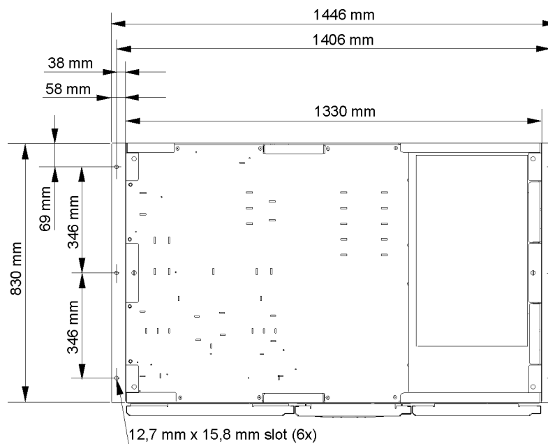
Рис. 2-5. Размеры ИБП (вид снизу с монтажными кронштейнами)
