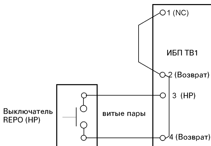
Рис. 3-13. Схема нормально разомкнутого подключения выключателя дистанционного аварийного отключения
