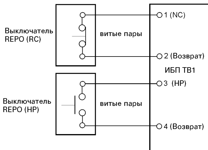
Рис. 3-14. Схема нормально замкнутого подключения выключателя дистанционного аварийного отключения
