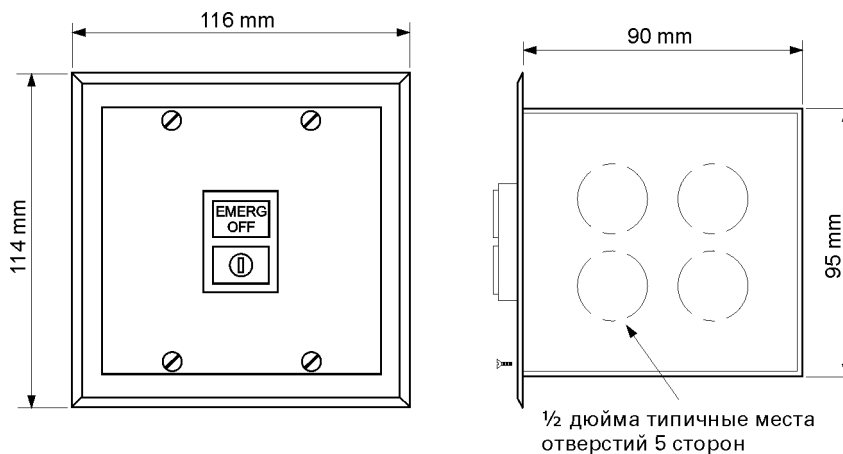
Рис. 2-7. Размеры порта удаленного аварийного отключения
