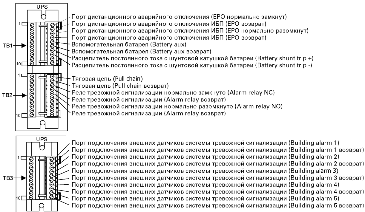
Рис. 3-8. Схема клемм подключения внешних устройств АА
