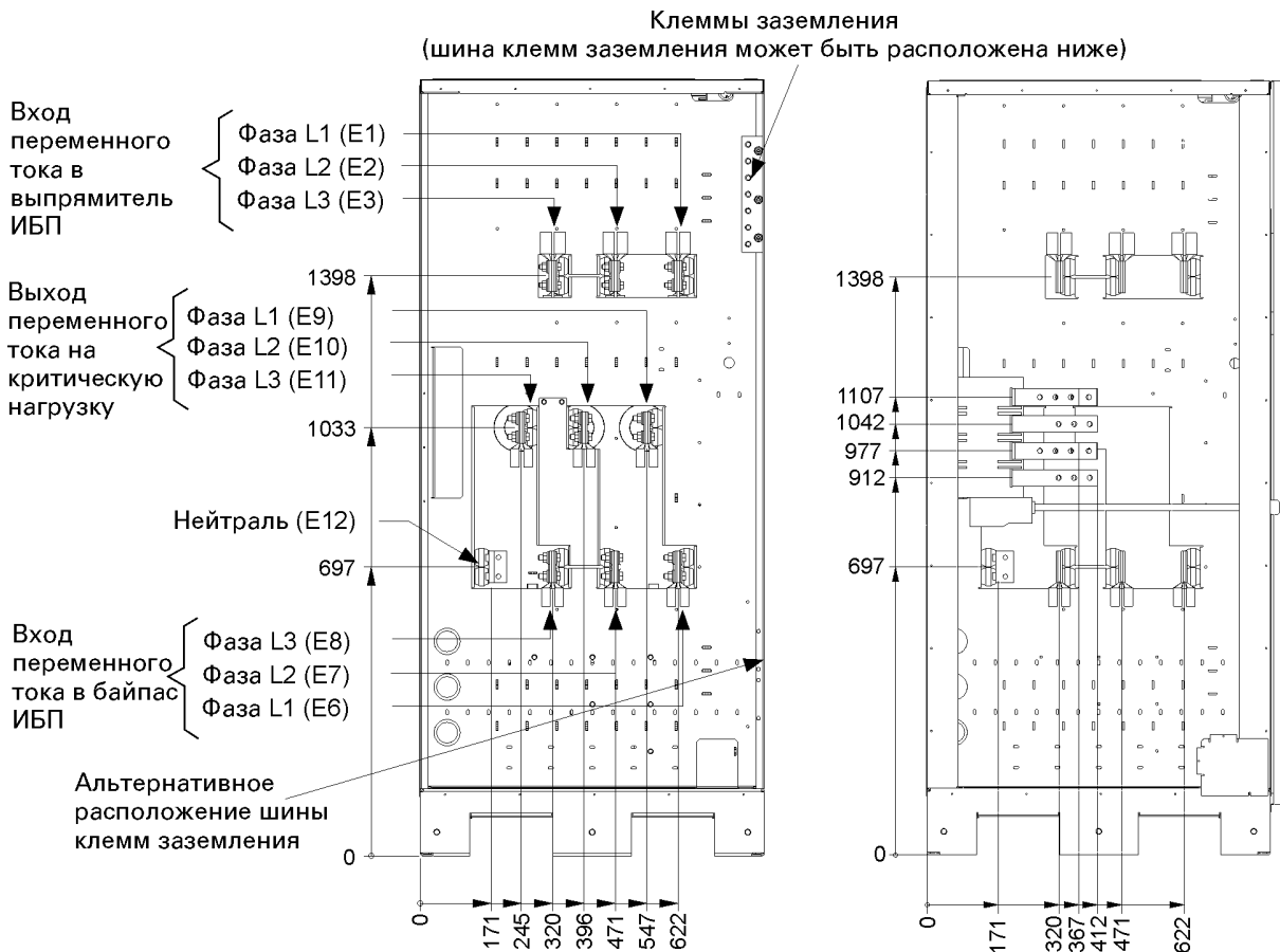
Рис. 3-5. Силовые выходы ИБП, схема АА
