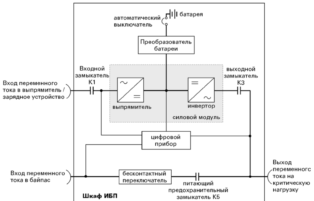
Рис. 4-1. Основные компоненты системы ИБП
