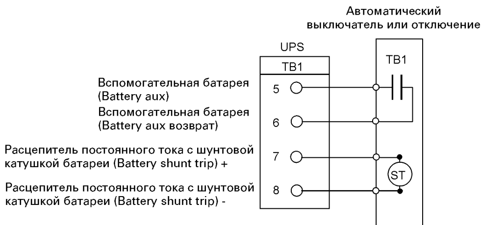
Рис. 3-10. Подключение сигнальных батарейных кабелей устройств к батареям
