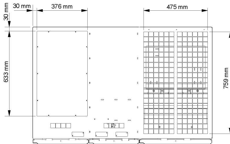
Рис. 2-3. Размеры ИБП (вид сверху)
