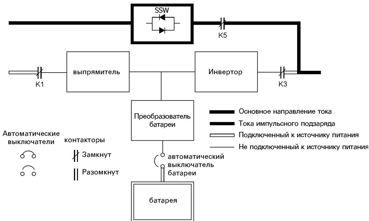
Рис. 4-3. Путь электрического тока через систему ИБП во время ее работы в режиме байпаса
