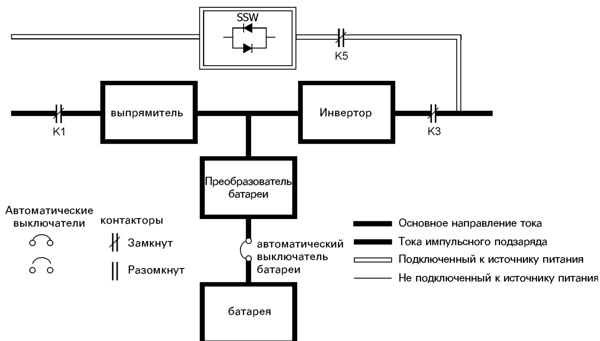
Рис. 4-2. Путь электрического тока через систему ИБП во время ее работы в нормальном режиме.
