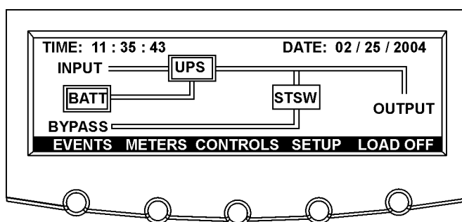
Рис. 5-4. Основное меню и мнемосхема (нормальный режим).
